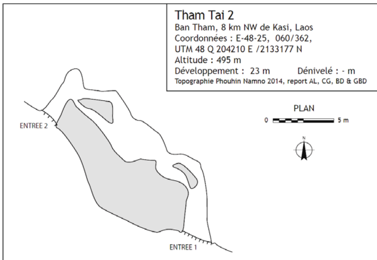
Figure 36 : Topographie de Tham Tai 2
