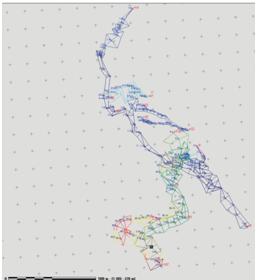
Figure 13 : Rendu Visual Topo des mesures faites à Tham Nam Fuang Tai. Z, l'altitude relative, est indiquée par une échelle de couleurs. On distingue trois niveaux principaux : niveau a (+150 m, rouge et jaune), porche fossile sud, porche fossile nord, galerie fossile ouest ; niveau b (+80, vert), galerie fossile centrale ; niveau c (+0, bleu), l'actif et ses galeries annexes.
