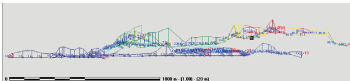
Figure 14 : Rendu Visual Topo en coupe. L'orientation des galeries est ici seulement fonction du sens de la topo et non de l'agencement réel de la cavité. On distingue les trois niveaux principaux de la cavité : niveau a (+150, rouge et jaune), niveau b (+80, vert) et niveau c (+0, bleu).
