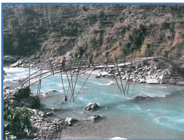
Pont de bambou sur la Bhote Khosi pour accéder à Kabre Khola
